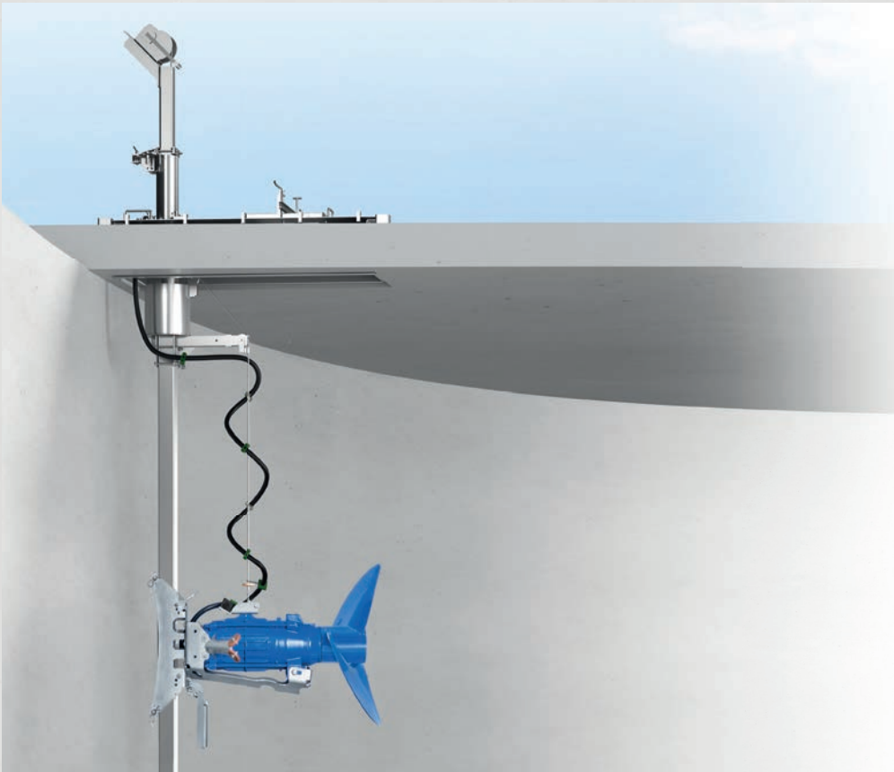
Illustration : EGR 4 (couverture de maintenance) avec GTWSB 204
